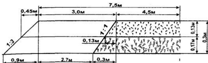
Рисунок 5. Схема поперечного профиля двухслойного щебеночного основания
