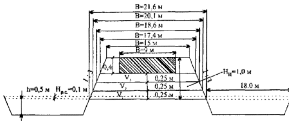
Рисунок 3. Конструкции земляного полотна в поперечном профиле Толщину срезаемого растительного слоя грунта устанавливают по
