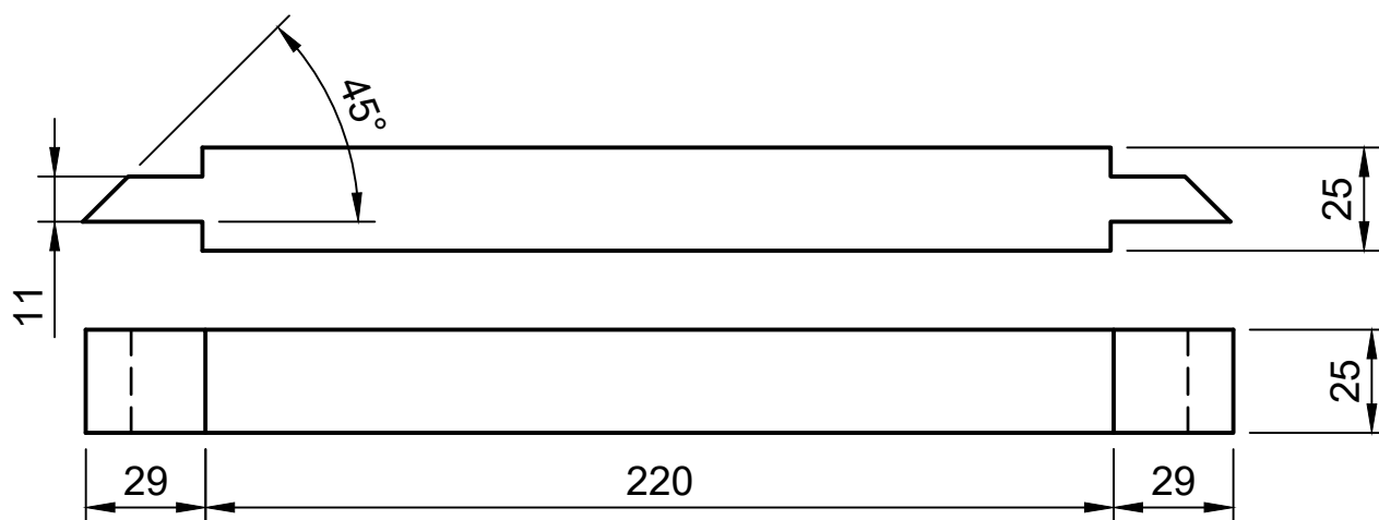
Проножка, 4 шт.
