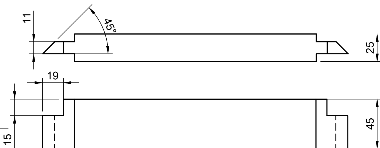
Проножка, 4 шт.
